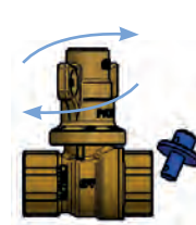
4 Girar el accionamiento hasta la posición de bloqueo deseada (bloqueo 10% apertura). / Rotate the handle until the required locked position (Lock in 10% opening).
