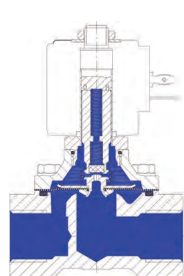
Bobina energizada / Coil energized Electroválvula abierta / Solenoid valve open
