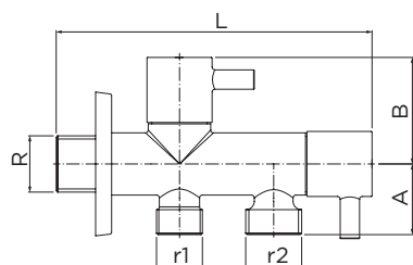
Ref.: 3109 04 Válvula de escuadra doble 1/2" - 3/8" Double angle valve 1/2" - 3/8"
