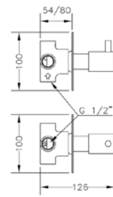
Ref.: 65114 30 45 66 Inversor cerámico 3 vías empotrado con placa cuadrada Built-in 3-way ceramic diverter with square plate
