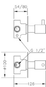
Ref.: 63114 30 45 66 Inversor cerámico 3 vías empotrado placa redonda Built-in 3 way ceramic diverter with round plate
