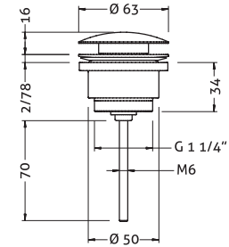
Ref.: 100211 45 Válvula universal click Luxe con y sin rebosadero Luxe universal click pop-up waste with and without overflow
