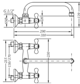
Ref.: 68555 09 45 66 Grupo mural fregadera 15 cm caño tubo alto 24 cm
