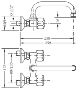
Ref.: 68195 11 45 66 Grupo mural fregadera 11 cm caño tubo alto 18 cm Wall sink mixer 11 cm high tube, 18 cm spout
