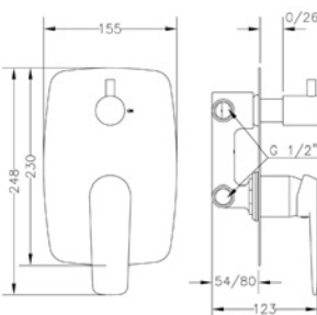
Ref.: 62117 31 45 66 Monomando empotrado con inversor cerámico 2 vías Built-in single lever mixer with 2 way ceramic diverter
