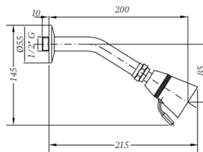
Ref.: 1698 45 00 Rociador ducha con brazo Wall shower arm and spray
