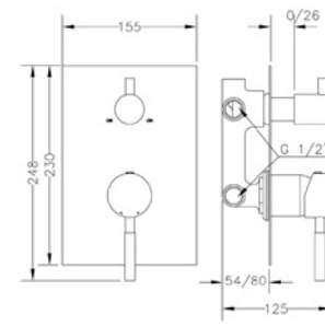
Ref.: 65118 18 45 66 Monomando empotrado con inversor cerámico 3 vías Built-in single lever mixer with 3-way ceramic diverter Box: 1 | Carton: 6 | Pallet: 108
