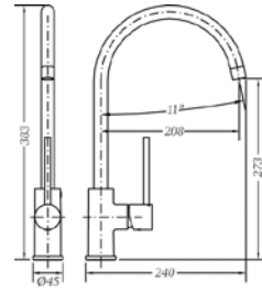
Ref.: FRT65401 Monomando de fregadera cartucho 25 apertura en frío Single lever sink mixer 25 cartridge cold start
