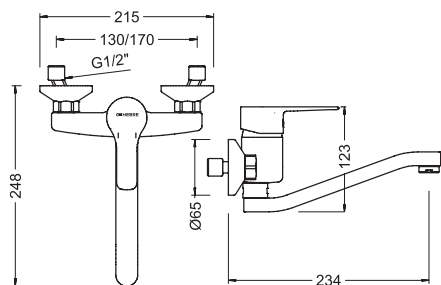
Ref.: 61196 28 45 66 Monomando de fregadera caño inferior elevado Wall single lever sink mixer low spout Box: 1 | Carton: 8 | Pallet: 192
