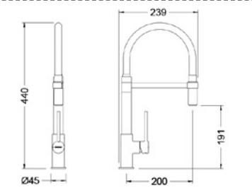
Ref.: 65219 18 45 66 Monomando de fregadera cartucho 25 apertura en frío Single lever sink mixer 25 cartridge cold start Box: 1 | Carton: 4 | Pallet: 48
