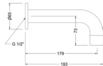
Ref.: 1668 41 Caño mural baño cilíndrico Negro Black Round wall bath spout
