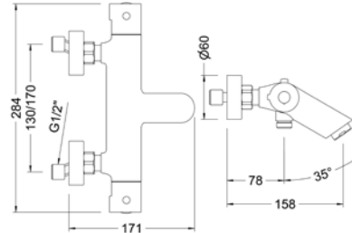
Ref.: 67102 14 45 67 Termostática baño Thermostatic bath mixer
