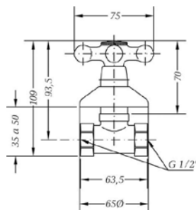
Ref.: 68590 09 43 66 Llave de paso 1/2" Bronce Bronze Stopcock 1/2"
