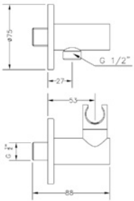
Ref.: 1633 04 Soporte de ducha orientable cilíndrico con toma 1/2" Orientable cylindrical shower holder with 1/2" connector Box: 1 | Carton: 75 | Pallet: 1800
