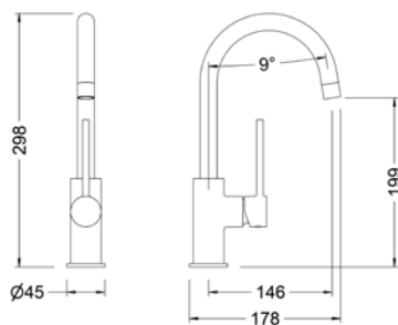
Ref.: 65138 18 45 66 Monomando de lavabo apertura en frío Single lever wash-basin tap cold start
