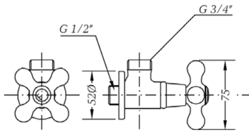
Ref.: 568575 45 Cuerpo grifo mural Wall body tap
