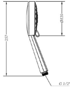
Ref.: DXT5 45 Mango de ducha T5 jets T5 jets handshower
