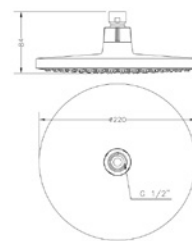
Ref.: R65112 41 Rociador D22 Oslo Black Oslo Black D22 shower head Box: 1 | Carton: 1
