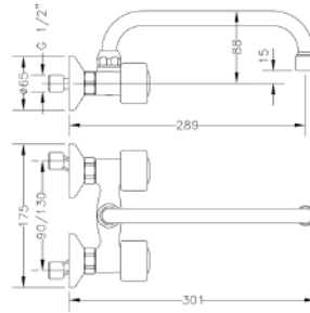
Ref.: 68196 11 45 66 Grupo mural fregadera 11 cm caño tubo alto 24 cm Wall sink mixer 11 cm high tube, 24 cm spout
