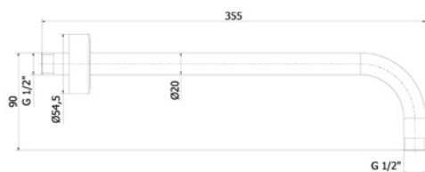
Ref.: B64113 41 Brazo pared redondo 35 cm negro Black round wall arm 35 cm
