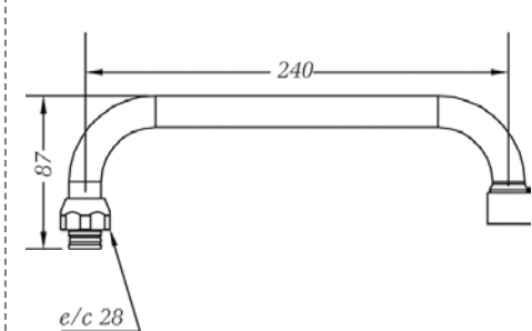
Ref.: 68902 45 Caño alto tubo 24 cm High pipe spout 24 cm
