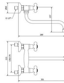
Ref.: 68560 09 45 66 Grupo mural fregadera 15 cm caño tubo bajo 24 cm
