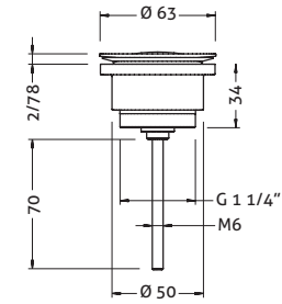
Ref.: 100205 45 Válvula universal click con y sin rebosadero Universal click pop-up waste with and without overflow
