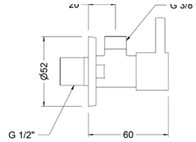
Ref.: 3104 04 Válvula de escuadra redonda 3/8" Round angle valve 3/8"
