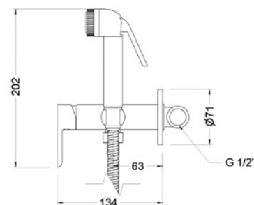
Ref.: 65144 19 45 66 Set mezclador sanitario de ducha con soporte Sanitary shower mixer set with support
