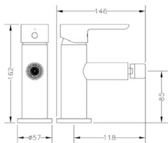
Ref.: 65140 19 45 66 Monomando de bidé Single lever bidet mixer
