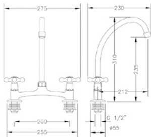
Ref.: 68545 09 45 66 Mezclador mesada 8" caño tubo
