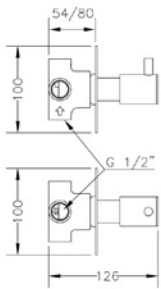
Ref.: 62114 30 45 66 Inversor cerámico 3 vías empotrado con placa ovalada Built-in 3 way ceramic diverter with oval plate
