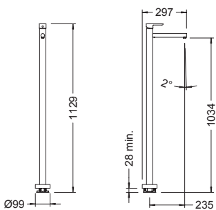
Ref.: 65139 19 45 66 Monomando de pie para lavabo Single-lever basin foot
