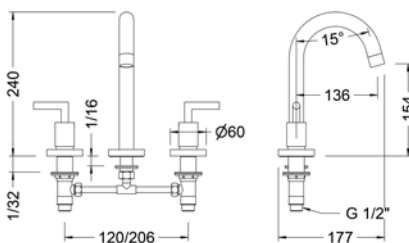
Ref.: 68124 12 45 66 Batería de lavabo caño cisne Widespread wash-basin mixer with swan pipe spout
