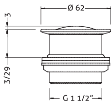
Ref.: 100208 45 Válvula universal click para bañera Click pop-up waste for bath
