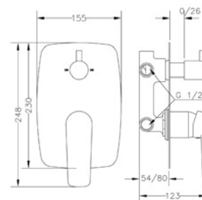
Ref.: 62118 31 45 66 Monomando empotrado con inversor cerámico 3 vías Built-in single lever mixer with 3 way ceramic diverter
