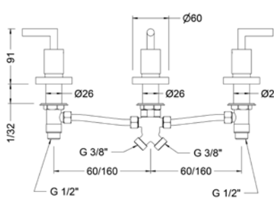
Ref.: 68113 12 45 66 Batería de baño con inversor Widespread bath mixer with diverter
