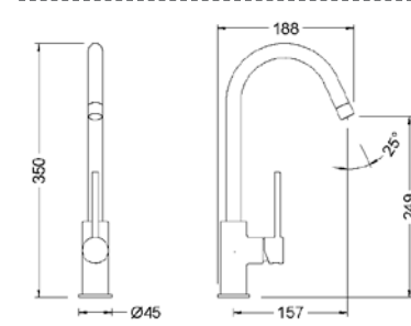
Ref.: 65403 18 40 66 Monomando de fregadera cartucho 25 apertura en frío Tau Blanca Tau White Single lever sink mixer 25 cartridge cold start
