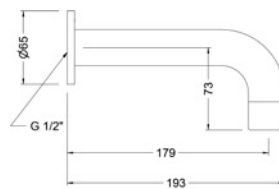
Ref.: 1668 45 Caño mural baño cilíndrico Round wall bath spout Box: 1 | Carton: 20 | Pallet: 240
