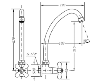
Ref.: 68575 09 45 66 Grifo fregadera mural caño tubo vertical
