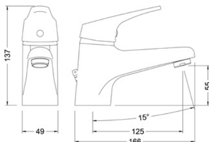
Ref.: 61130 22 45 66 Monomando de lavabo Plus Single lever Plus wash-basin mixer
