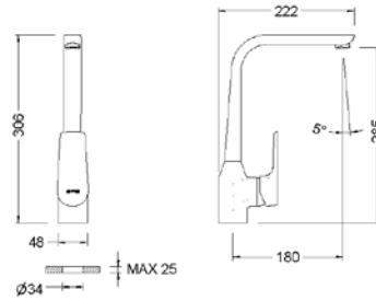
Ref.: 64201 32 45 66 Monomando de fregadera Korál Korál Single lever sink mixer
