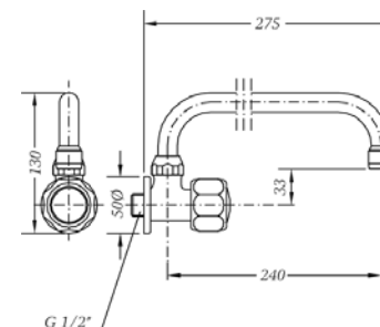
Ref.: 68093 11 45 66 Grifo mural fregadera caño tubo alto 24 cm
