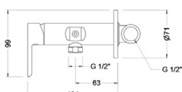
Ref.: 65144 19 41 67 Mezclador sanitario de ducha con soporte Negro Black Sanitary shower mixer with support
