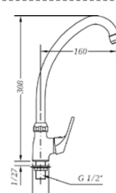
Ref.: 1009 04 Grifo fregadera 1 agua cartucho 25 One-water sink tap 25 cartridge Box: 1 | Carton: 30 | Pallet: 540
