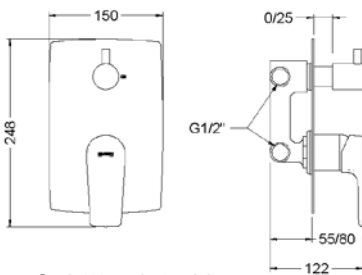
Ref.: 64117 32 45 66 Monomando empotrado con inversor cerámico 2 vías Built-in single lever mixer with 2-way ceramic diverter
