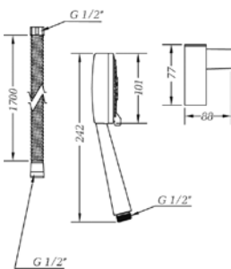
Ref.: 100698 45 Kit de ducha Kenjo, flexo, soporte y ducha 3 jets
