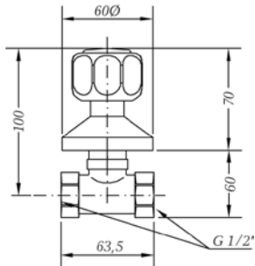
Ref.: 68170 11 45 66 Llave de paso 1/2" Stopcock 1/2"
