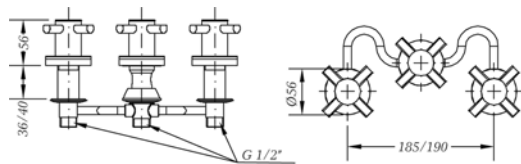
Ref.: 68142 08 45 66 Batería de bidé con transmisión Widespread bidet mixer with transmission
