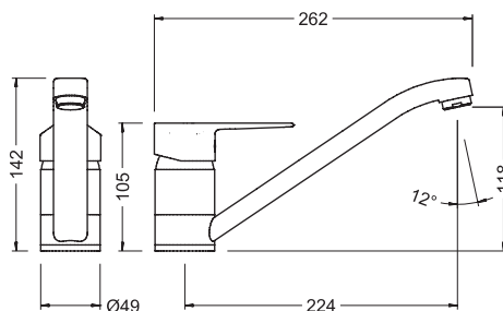
Ref.: 61200 28 45 66 Monomando de fregadera Single lever sink mixer Box: 1 | Carton: 9 | Pallet: 216
