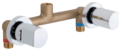
Grupo ducha empotrado 8" Built-in 8" shower mixer Ref.: 68115 07 45 66
