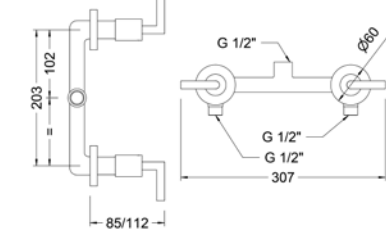
Ref.: 68115 07 45 66 Grupo ducha empotrado 8" Built-in 8" shower mixer
