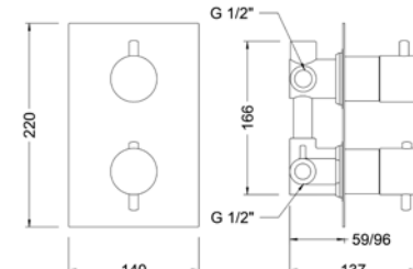
Ref.: 64111 14 45 67 Termostática empotrada 3 vías Built-in 3-way thermostatic
