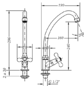
Ref.: 68585 09 45 66 Grifo fregadera encimera caño tubo vertical
