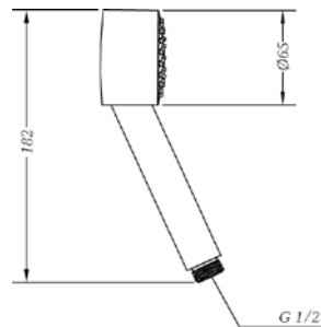
Ref.: 100197 45 00 Mango de ducha C1 jet C1 jet handshower
