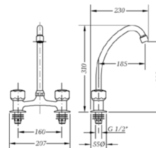
Ref.: 68194 11 45 66 Mezclador mesada 6" caño tubo
