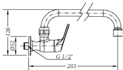
Ref.: 1008 04 Grifo mural con tubo 24 cm 1 agua cartucho 25 One-water wall sink tap spout 24 cm 25 cartridge Box: 1 | Carton: 30 | Pallet: 540
