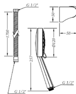
Ref.: 100699 45 Kit de ducha Tau, flexo, soporte y ducha 5 jets
