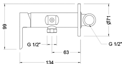
Ref.: 65144 19 45 67 Mezclador sanitario de ducha con soporte Sanitary shower mixer with support
