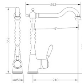
Ref.: 68201 39 45 66 Monomando de fregadera cromo Chromed sink mixer
