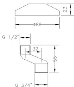
Ref.: 100122 45 Conjunto florón y excéntricas gigantes Giant scutcheon and eccentric set
