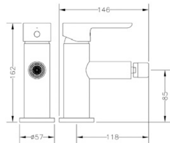
Ref.: 65140 19 41 66 Monomando de bidé Single lever bidet mixer
