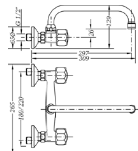
Ref.: 68104 11 45 66 Grupo mural fregadera 20 cm caño tubo alto 24 cm
