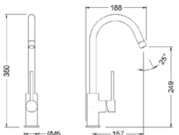
Ref.: 65403 18 41 66 Monomando de fregadera cartucho 25 apertura en frío Tau Black Tau Black Single lever sink mixer 25 cartridge cold start
