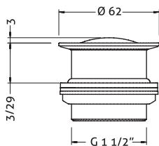
Ref.: 100208 43 Válvula universal click para bañera Bronce Bronze Click pop-up waste for bath
