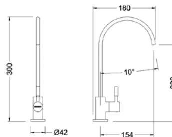
Ref.: 65700 18 45 66 Grifo de 1 vía One way tap Box: 1 | Carton: 14 | Pallet: 252
