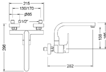
Ref.: 64192 32 45 66 Monomando de fregadera mural Korál Korál Wall single lever sink mixer
