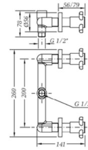
Ref.: 68115 08 45 66 Grupo ducha empotrado 8" Built-in 8" shower mixer
