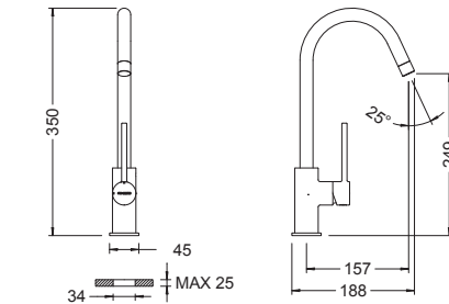
Ref.: 65403 18 44 66 Monomando de fregadera Tau acabado Acero Inoxidable cartucho 25 apertura en frío Tau Stainless steel finish single lever sink mixer 25 cartridge cold start
