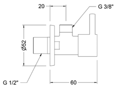
Ref.: 3110 03 41 Válvula de escuadra redonda 3/8" Negro Black Round angle valve 3/8"
