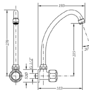
Ref.: 68083 11 45 66 Grifo fregadera mural caño tubo vertical
