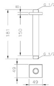
Ref.: 1672 45 Brazo a techo cuadrado 15 cm Square roof arm 15 cm Box: 1 | Carton: 20 | Pallet: 800
