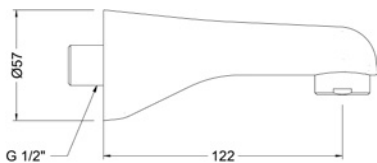
Ref.: 1667 45 Caño mural baño fundido Casted wall bath spout Box: 1 | Carton: 60 | Pallet: 1080
