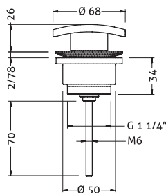
Ref.: 100204 45 Válvula universal click Kenjo con y sin rebosadero Kenjo universal click pop-up waste with and without overflow
