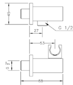
Ref.: 1649 04 Soporte de ducha orientable cuadrado con toma 1/2" Orientable square shower holder with 1/2" connector Box: 1 | Carton: 50 | Pallet: 1600
