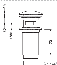
Ref.: 100210 45 Válvula universal click lavabo y bidé click doble función Double function click pop-up waste for basin and bidet
