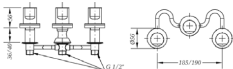
Ref.: 68142 07 45 66 Batería de bidé con transmisión Widespread bidet mixer with transmission
