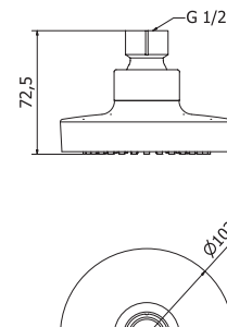
Ref.: 1155 04 Rociador cilíndrico 10cm Cylindrical shower head 10cm
