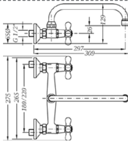
Ref.: 68565 09 45 66 Grupo mural fregadera 20 cm caño tubo alto 24 cm
