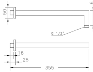
Ref.: B63113 26 Brazo pared cuadrado 35 cm Square wall arm 35 cm
