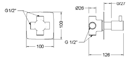
Ref.: 64114 30 45 66 Inversor cerámico 3 vías empotrado Built-in 3-way ceramic diverter
