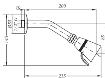
Ref.: 1698 45 00 Rociador ducha con brazo Wall shower arm and spray Box: 1 | Carton: 15 | Pallet: 480
