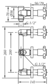
Ref.: 68116 08 45 66 Grupo ducha empotrado 8" con inversor Built-in 8" bath mixer with diverter
