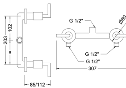
Ref.: 68115 12 45 66 Grupo ducha empotrado 8" Built-in 8" shower mixer
