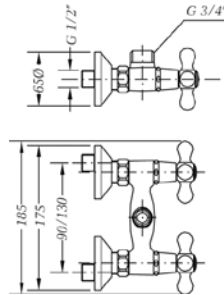
Ref.: 568550 45 Cuerpo grupo mural 11 cm Wall body mixer 11 cm
