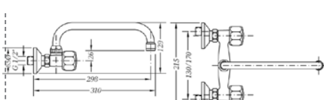
Ref.: 68193 11 45 66 Grupo mural fregadera 15 cm caño tubo alto 24 cm
