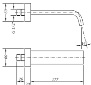
Ref.: 1674 45 Caño mural baño cuadrado Square wall bath spout Box: 1 | Carton: 24 | Pallet: 720
