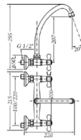
Ref.: 68570 09 45 66 Grupo mural fregadera 20 cm caño tubo alto vertical
