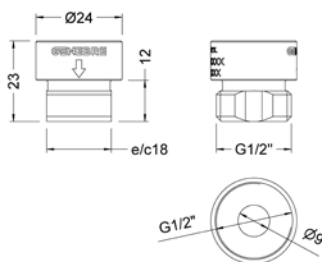
Ref.: 9908 0300 - 9908 0307 Conector 1/2\"/>
