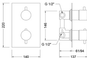
Ref.: 64114 14 45 67 Termostática empotrada 2 vías Built-in 2-way thermostatic mixer
