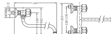
Ref.: 68197 11 45 66 Grupo mural fregadera 15 cm caño tubo bajo 24 cm
