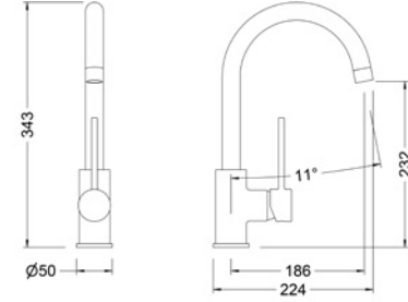
Ref.: FRT65402 Monomando de fregadera cartucho 35 apertura en frío Single lever sink mixer 35 cartridge cold start Box: 1 | Carton: 8 | Pallet: 96
