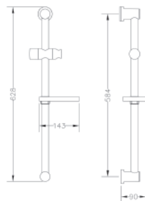
Ref.: 1638 45 Barra ducha redonda Round shower bar
