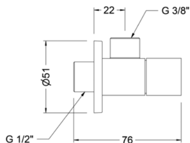
Ref.: 3106 05 Válvula de escuadra cuadrada 1/2" Square angle valve 1/2"
