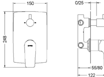
Ref.: 64118 32 45 66 Monomando empotrado con inversor cerámico 3 vías Built-in single lever mixer with 3-way ceramic diverter
