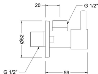
Ref.: 3110 04 41 Válvula de escuadra redonda 1/2" Negro Black Round angle valve 1/2"
