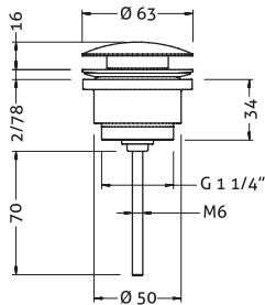
Ref.: 100211 41 Válvula universal click Luxe con y sin rebosadero Negro Black luxe universal click pop-up waste with and without overflow
