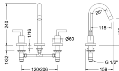
Ref.: 68125 12 45 66 Batería de lavabo caño inclinado Widespread wash-basin mixer with sloping pipe spout
