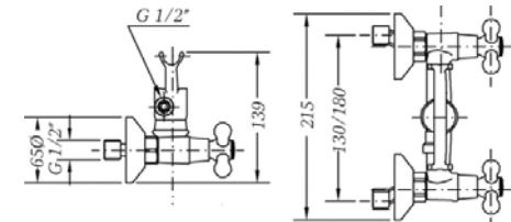
Ref.: 68531 09 43 66 Mezclador de ducha bronce con kit Bronze shower mixer with kit
