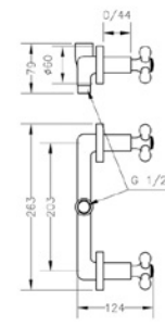
Ref.: 68535 09 45 66 Grupo ducha empotrado 8" Built-in 8" shower mixer
