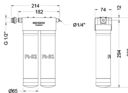
Ref.: FT01 Kit ultrafiltración Ultrafiltration kit
