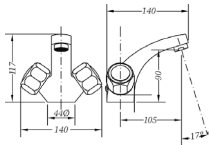
Ref.: 68130 11 45 66 Monobloc de lavabo Wash-basin mixer
