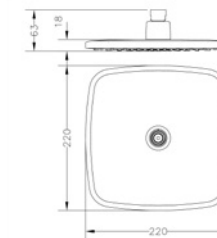
Ref.: R63112 08 Rociador D22 ovalado Oval D22 shower sprayer Box: 1 | Carton: 24 | Pallet: 192
