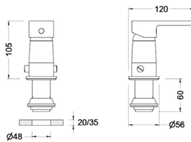
Ref.: 65142 19 41 66 Monomando de bidé con transmisión Single lever bidet mixer with diverter
