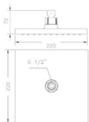
Ref.: R63112 26 Rociador cuadrado 22 cm Square shower head 22 cm Box: 1 | Carton: 24 | Pallet: 144
