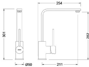
Ref.: 65404 18 45 66 Monomando de fregadera cartucho 35 apertura en frío Single lever sink mixer 35 cartridge cold start Box: 1 | Carton: 8 | Pallet: 96
