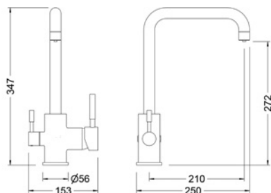
Ref.: 65702 18 45 66 Monomando de fregadera 3 vías apertura en frío Single lever 3-way sink mixer cold start Box: 1 | Carton: 4 | Pallet: 96
