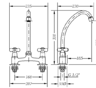
Ref.: 68194 09 45 66 Mezclador mesada 16 cm caño tubo
