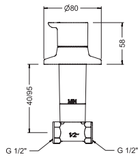
Ref.: 60170 41 45 66 Llave de paso 1/2" 1/2" Stopcock
