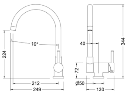
Ref.: 65900 18 45 66 Monomando de fregadera abatible cartucho 35 apertura en frío Single lever folding sink mixer 35 cartridge cold start Box: 1 | Carton: 8 | Pallet: 96
