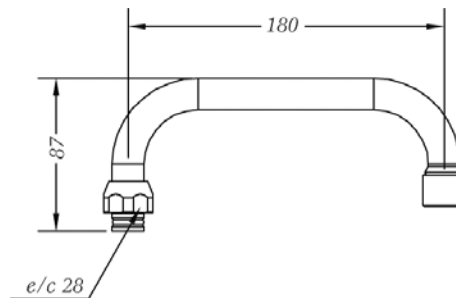
Ref.: 68901 45 Caño alto tubo 18 cm High pipe spout 18 cm
