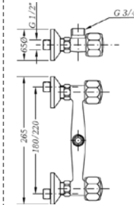
Ref.: 568104 45 Cuerpo grupo mural 20 cm Wall body mixer 20 cm
