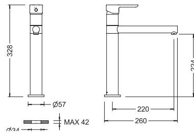
Ref.: 65200 19 45 66 Monomando de fregadera Single lever sink mixer
