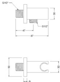
Ref.: 1635 04 Soporte de ducha cuadrado con toma 1/2" Square shower holder with 1/2" connector Box: 1 | Carton: 1
