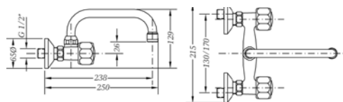
Ref.: 68190 11 45 66 Grupo mural fregadera 15 cm caño tubo alto 18 cm
