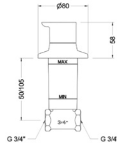
Ref.: 60171 41 45 66 Llave de paso 3/4" 3/4" Stopcock
