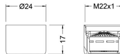
Ref.: 9908 0316 - 9908 0321 Aireador antical H22x1 baja presión F22x1 Anti-lime low pressure aerator
