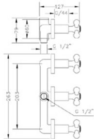
Ref.: 68527 09 45 66 Grupo baño empotrado 8" con inversor Built-in 8" bath mixer with diverter
