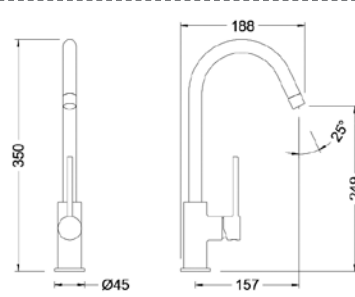
Ref.: 65403 18 45 66 Monomando de fregadera cartucho 25 apertura en frío Single lever sink mixer 25 cartridge cold start Box: 1 | Carton: 8 | Pallet: 96
