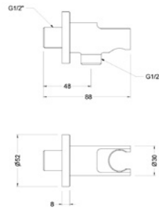
Ref.: 1634 04 Soporte de ducha cilíndrico con toma 1/2" Cylindrical shower holder with 1/2" connector Box: 1 | Carton: 1
