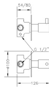
Ref.: 63114 30 45 66 Inversor cerámico 3 vías empotrado placa redonda Built-in 3 way ceramic diverter with round plate
