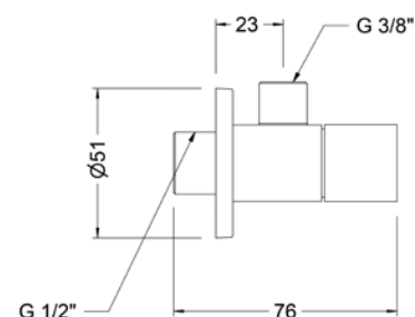
Ref.: 3106 04 Válvula de escuadra cuadrada 3/8" Square angle valve 3/8"
