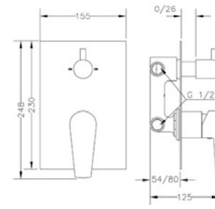
Ref.: 64117 04 45 66 Monomando empotrado con inversor cerámico 2 vías Built-in single lever mixer with 2-way ceramic diverter
