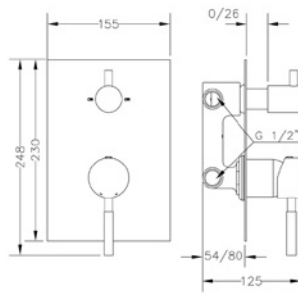
Ref.: 65117 18 45 66 Monomando empotrado con inversor cerámico 2 vías Built-in single lever mixer with 2-way ceramic diverter Box: 1 | Carton: 6 | Pallet: 108
