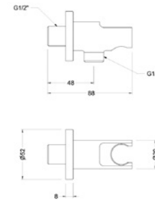
Ref.: 1946 41 Soporte de ducha cilíndrico con toma 1/2" Negro Black Cylindrical shower holder with 1/2" connector Box: 1 | Carton: 1
