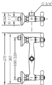
Ref.: 568565 45 Cuerpo grupo mural 20 cm Wall body mixer 20 cm
