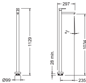
Ref.: 65139 19 41 66 Monomando de pie para lavabo negro Black single-lever basin foot
