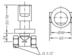
Ref.: 68170 07 45 66 Llave de paso 1/2" Stopcock 1/2"
