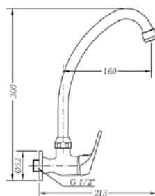
Ref.: 1005 04 Grifo mural con tubo alto 1 agua cartucho 25 One-water wall sink tap high spout 25 cartridge Box: 1 | Carton: 30 | Pallet: 540
