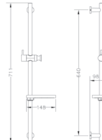
Ref.: 1639 45 Barra ducha metálica Round shower bar Metallic
