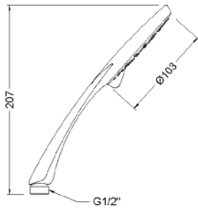
Ref.: 9908 0284 Mango de ducha 3 jets negro Black 3 jets hand shower
