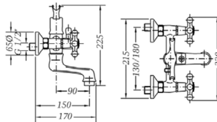
Ref.: 68526 09 43 66 Mezclador de baño bronce con kit Bronze bath mixer with kit
