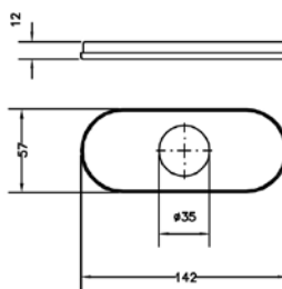
Ref.: P130 Placa adaptadora 4" 4" adaptor plate
