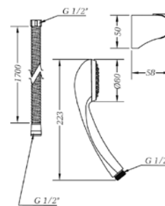
Ref.: 100697 45 Kit de ducha GE2, flexo, soporte y ducha 1 jet
