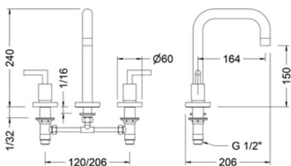
Ref.: 68120 12 45 66 Batería de lavabo caño recto Widespread wash-basin mixer with straight pipe spout
