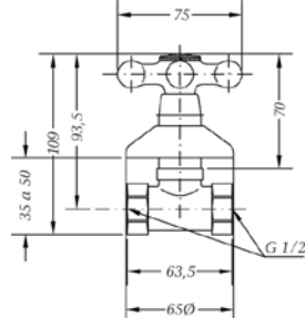
Ref.: 68590 09 45 66 Llave de paso 1/2" Stopcock 1/2"
