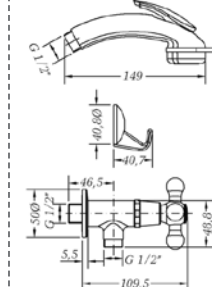
Ref.: 68001 09 45 66 Grifo de bidé con teleducha Bidet tap with shower
