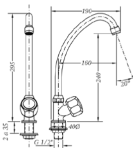
Ref.: 68003 11 45 66 Grifo fregadera encimera caño tubo vertical
