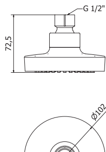
Ref.: 1155 04 Rociador cilíndrico 10cm Cylindrical shower head 10cm Box: 1 | Carton: 48 | Pallet: 864
