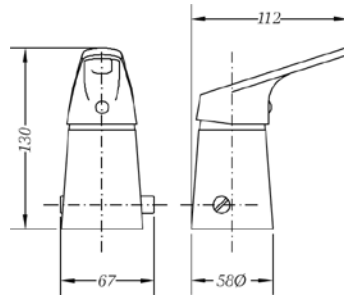
Ref.: 61142 22 45 66 Monomando de bidé con transmisión Single lever bidet mixer with diverter Box: 1 | Carton: 12 | Pallet: 216
