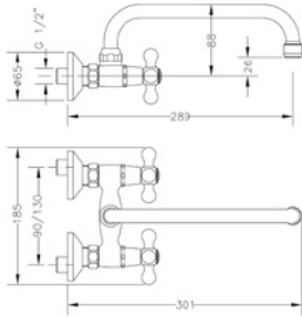
Ref.: 68196 09 45 66 Grupo mural fregadera 11 cm caño tubo alto 24 cm
