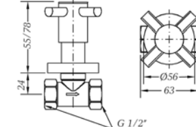
Ref.: 68170 08 45 66 Llave de paso 1/2" Stopcock 1/2"
