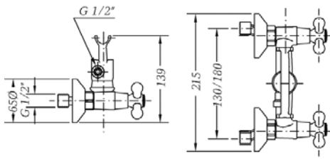
Ref.: 68531 09 45 66 Mezclador de ducha cromo con kit Chromed shower mixer with kit
