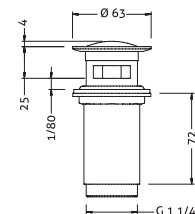
Ref.: 100209 45 Válvula universal click lavabo y bidé click doble función double function click pop-up waste for basin and bidet
