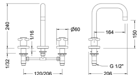
Ref.: 68120 08 45 66 Batería de lavabo caño recto Widespread wash-basin mixer with straight pipe spout
