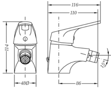
Ref.: 60140 22 45 66 Monomando de bidé Single lever bidet mixer Box: 1 | Carton: 8 | Pallet: 480
