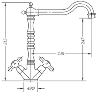
Ref.: 68595 09 45 66 Monobloc de fregadera cromo Chromed sink mixer
