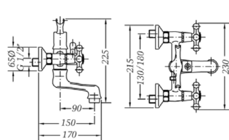
Ref.: 68526 09 45 66 Mezclador de baño cromo con kit Chromed bath mixer with kit
