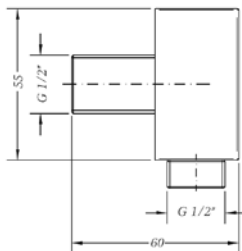
Ref.: 1679 04 Toma ducha mural cuadrada Square wall connector Box: 1 | Carton: 40 | Pallet: 2304
