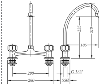
Ref.: 68199 11 45 66 Mezclador mesada 8" caño tubo 8" deck mixer with swan neck spout
