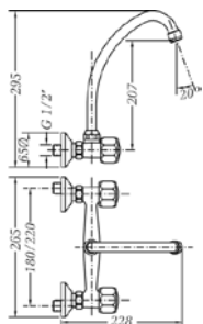
Ref.: 68103 11 45 66 Grupo mural fregadera 20 cm caño tubo alto vertical
